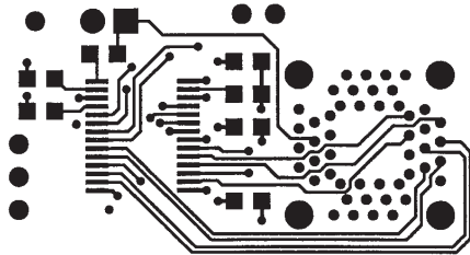
TOP LAYER
