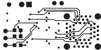
BOTTOM LAYER
